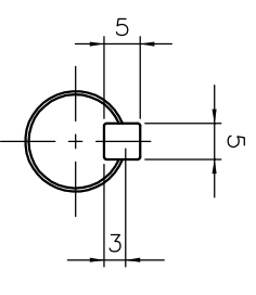
<축단 치수 상세도>
