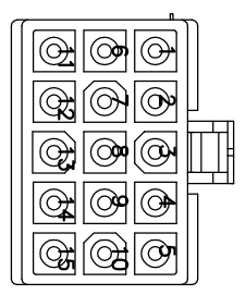
Plug 사양:172171-1 (AMP)
