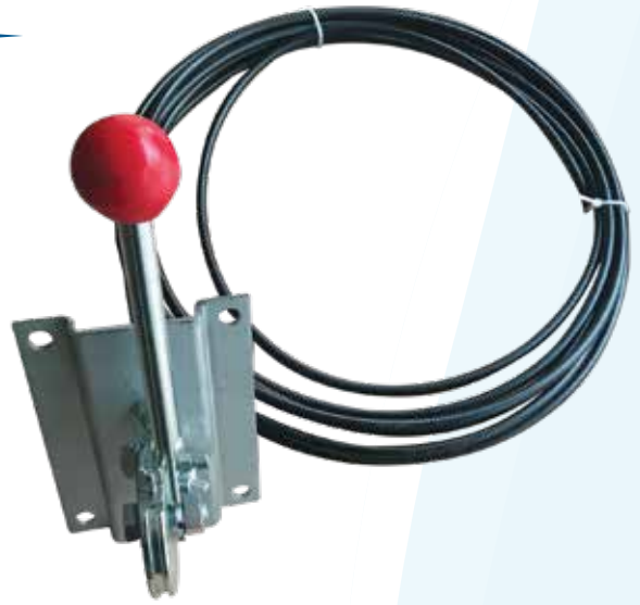
Manuel fren açtırma kolu ve çelik tel 7m. Manual brake relase device and steel wire 7m.
